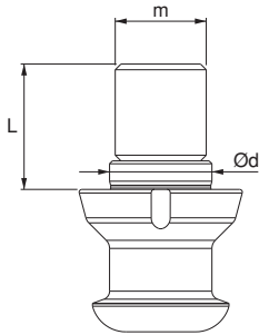
Ürün Nr. 1065 Çektirme Civatası
